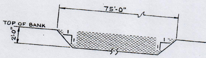
SECTION "B-B" SCALE: 1/4" = 1'-0"
