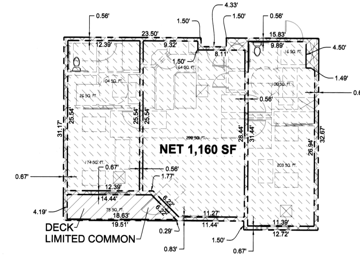
TYPE G (2 BED ADA)
